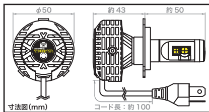
寸法図(mm)
