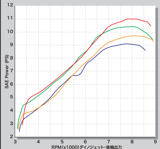
Sステージボアアップキット138cc(カムシャフト付属)
