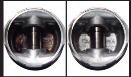
1000kmテスト結果 ピストン/ピストンピン (左:ノーマルポンプ 右:スーパーオイルポンプ)
