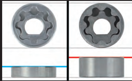
トロコイドローター厚み比較 (左:ノーマルポンプ 右:スーパーオイルポンプ)
