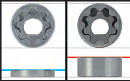
トロコイドローター厚み比較 (左:ノーマルポンプ 右:スーパーオイルポンプ)
