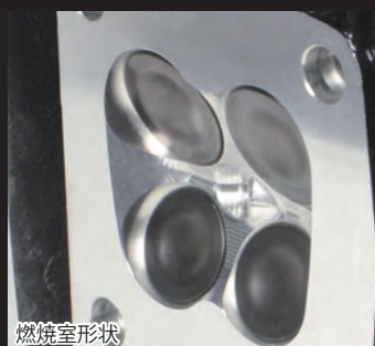
燃焼室形状
