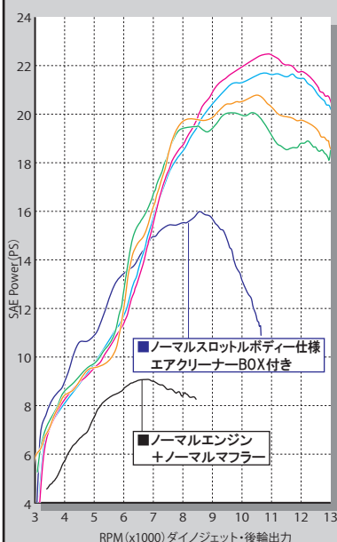
スーパーヘッド4V+R コンボキット181cc (ビッグスロットルボディー付属) (01-05-0212)
