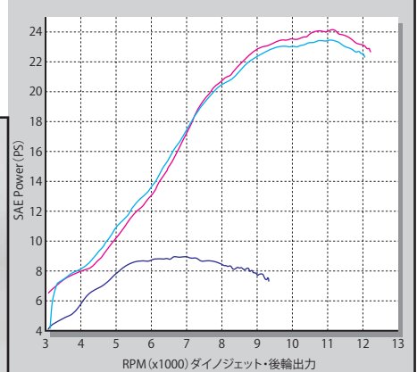
テスト車両:モンキー125(JB02) スーパーヘッド4V+Rコンプリートエンジン(ビッグスロットルボディ) +FICON TYPE-X(インジェクションコントローラー) +テーパーコーンマフラー ■15-15Dオプショナルカムシャフト ■10-10D付属カムシャフト ■ノーマルエンジン+ノーマルマフラー
