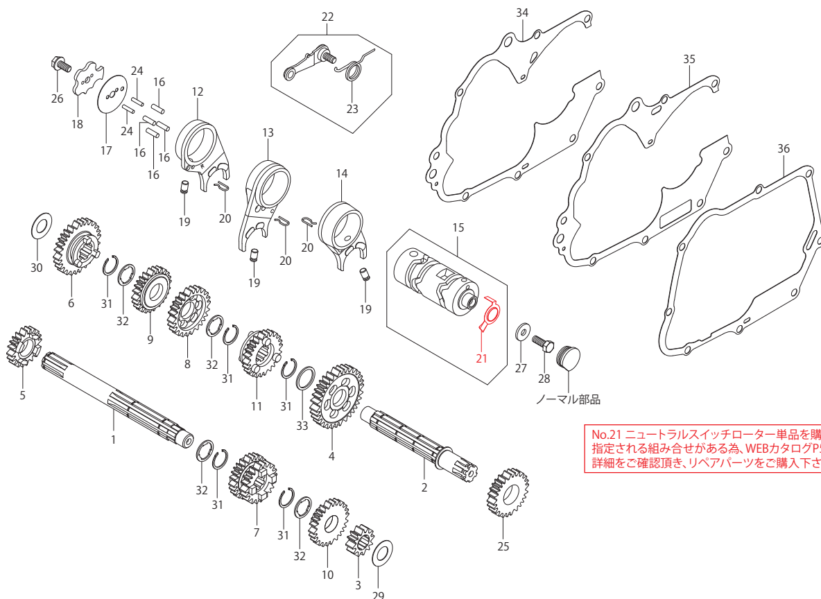
■乾式/DRY用 SS5速クロスミッション ストリート 02-04-0204 ¥80,300(税込) リペアパーツ
