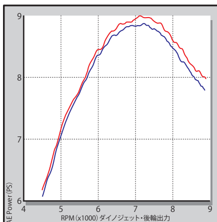
ビッグスロットルボディーキット Φ28
