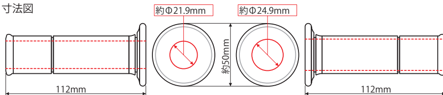
寸法図
