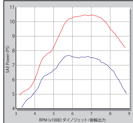
テスト車両:CT125 (JA55) ■eステージαポアアップキット143cc+スポーツマフラー ■ノーマルエンジン+ノーマルマフラー
