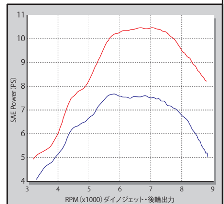
テスト車両:CT125 (JA55) ■eステージαボアアップキット143cc+スポーツマフラー ■ノーマルエンジン+ノーマルマフラー
