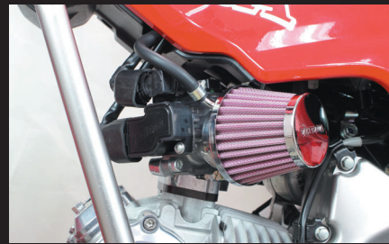
装着写真(SP武川製ビッグスロットルボディー)
