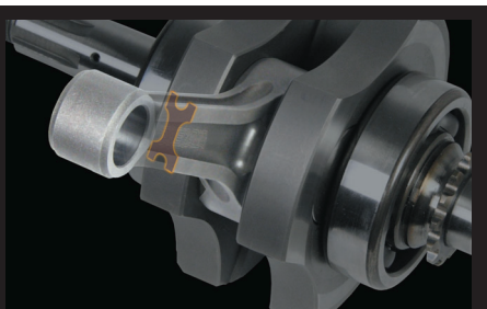
X断面形状コンロッド採用
