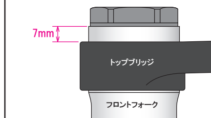
フロントフォーク突き出し詳細図
