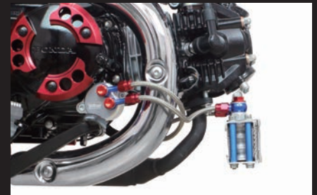
装着写真 (07-07-0452)
