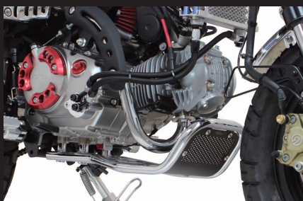
装着写真(モンキー125/クロムメッキ)
