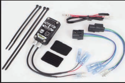
05-06-0065 (製品構成)
