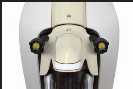
05-08-0673 (2灯仕様) 装着写真
