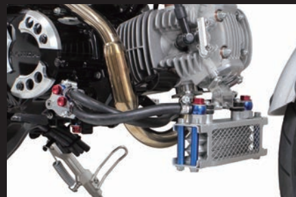
3フィン4オイルライン装着
