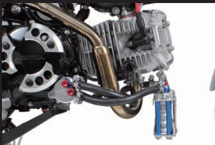
4フィン5オイルライン装着
