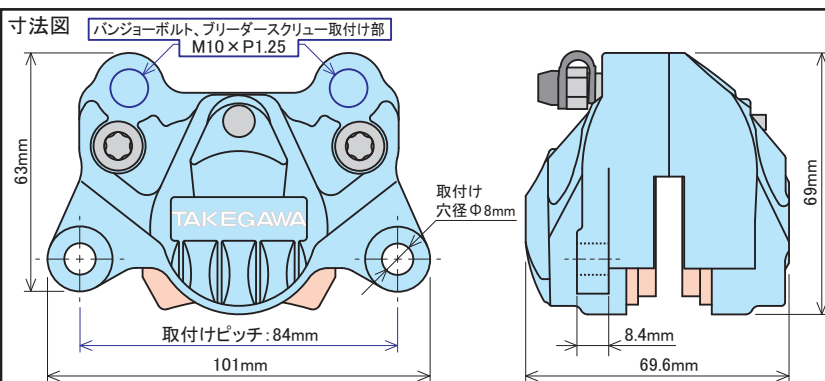
モンキー125 (JB05) ABS車 SP武川製キャリパーブラケット同時装着 (純正ブレーキホース/ディスクローター)
