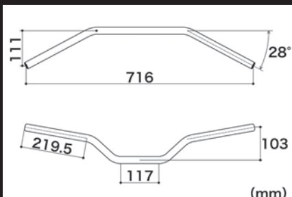
ハンドルパイプ寸法図
