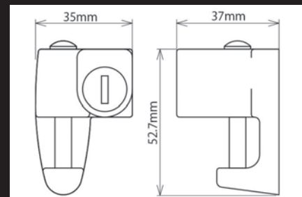
ホルダー本体寸法図
