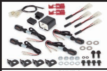
05-08-0715 製品構成
