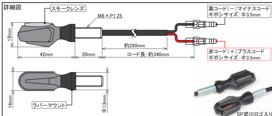
05-08-0713 製品構成 (2個セット)
