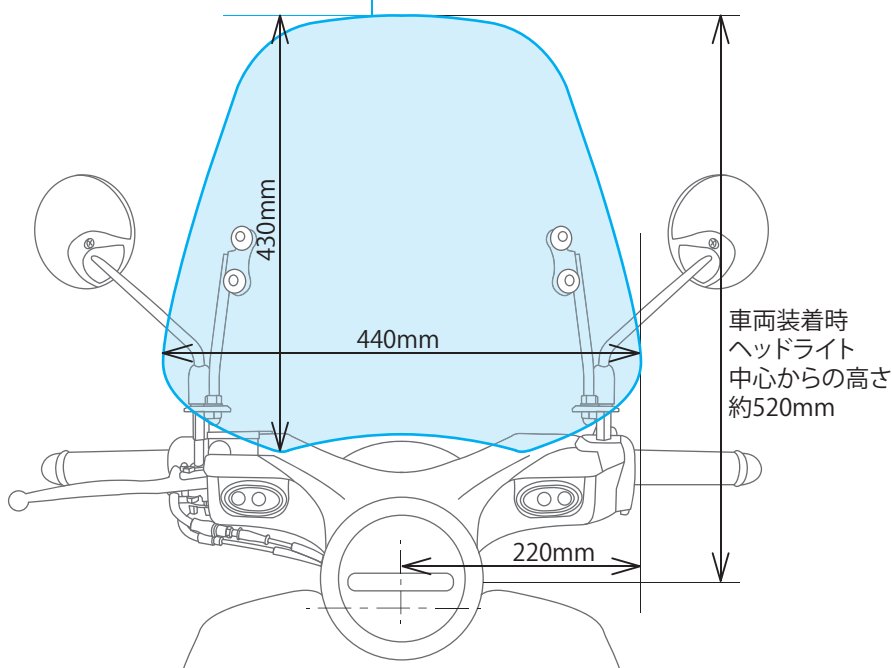
詳細図
