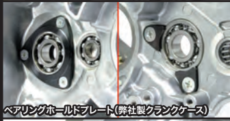
ベアリングホルドプレート(弊社製クランクケース)
