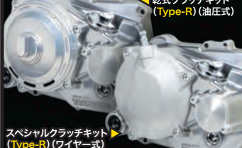
乾式クラッチキット (Type-R) (油圧式)
