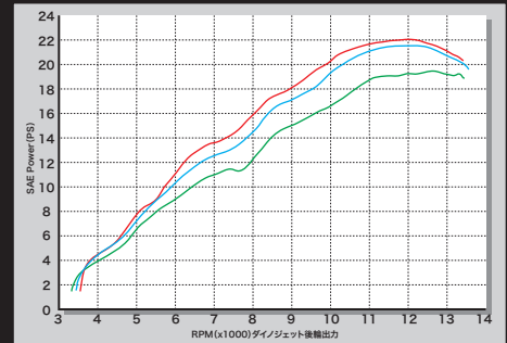
スーパーヘッド4V+R コンプリートエンジン +KEIHIN PE28キャブレター+レーシングマフラー ■148cc(25/30Dカムシャフト) ■138cc(20/25Dカムシャフト) ■123cc(20/25Dカムシャフト) ※実走行とは異なります。参考データとしてご覧ください。
