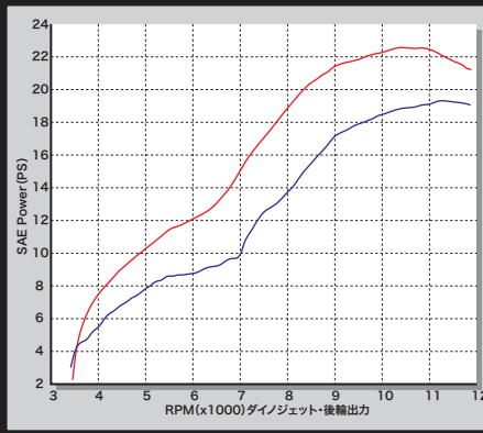
スーパーヘッド4V+R(1カム4バルブ) アルミダイカスト製バフ研磨クリア塗装クラッチカバー (ワイヤー式)
