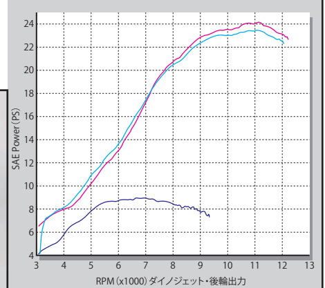
テスト車両：モンキー125 (JB02) スーパーヘッド4V+Rコンプリートエンジン(ビッグスロットルボディ) +FIコンTYPE-X(インジェクションコントローラー) +テーパーコーンマフラー ■15-15Dオープンジョナルカムシャフト ■10-10D付属カムシャフト ■ノーマルエンジン+ノーマルマフラー
