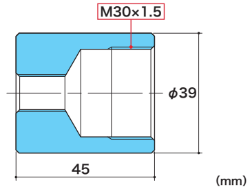
フライホイールプーラー詳細図
