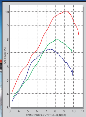
テスト車:クロスカブ (JA10) ■ハイパーSステージボアアップキット125cc + スポーツマフラー ■ノーマルエンジン + スポーツマフラー ■ノーマルエンジン + ノーマルマフラー
