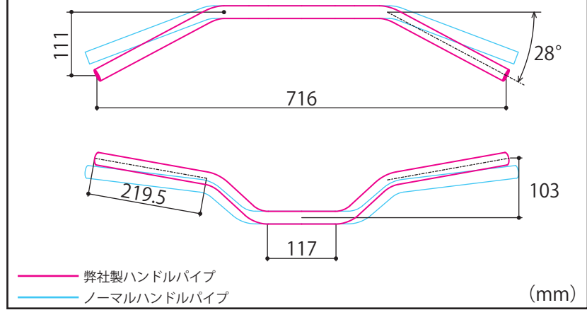
寸法図(ノーマルハンドルとの比較)
