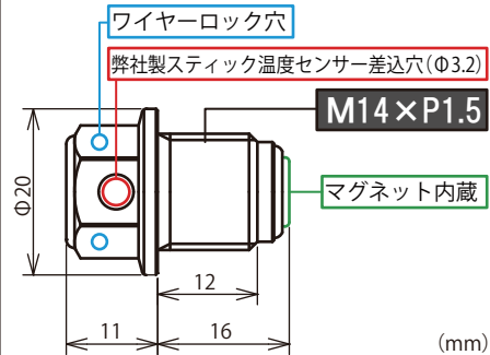
詳細図
