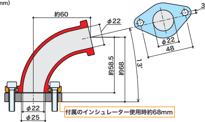
マニホールド詳細図 (mm)
