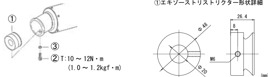
①エキゾーストリストラクター形状詳細
