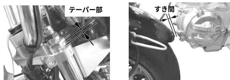
フロントフォークと使用タイヤの関係 148cc
