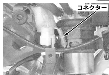
2Pカブラ
