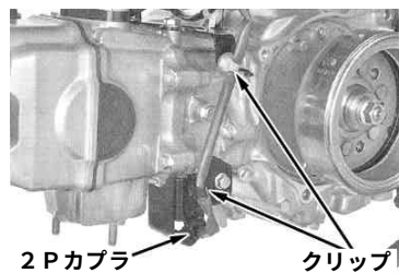
コネクター
