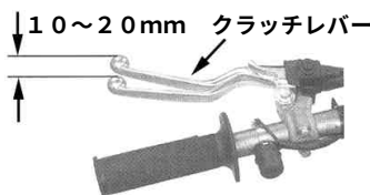
クラッチの遊び : クラッチレバー先端で 10 ~ 20 mm
