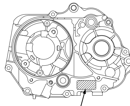
エンジンNo打刻位置 4SMS-200**
