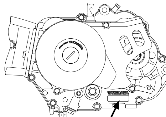
エンジン打刻位置 2SMS-20001～
