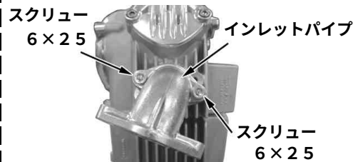
スクリュー 6×25
