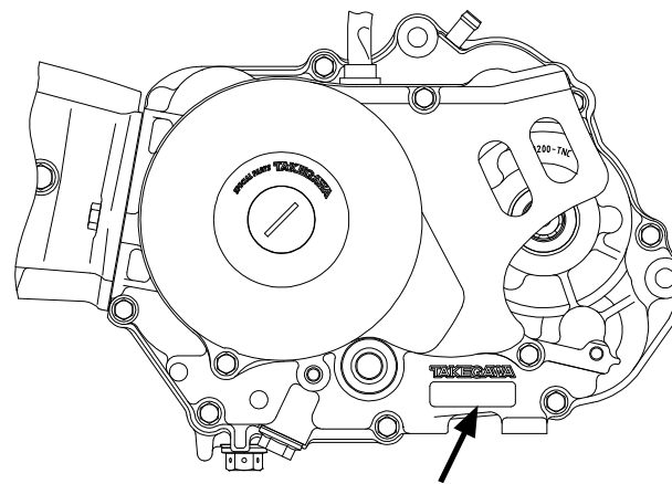
エンジン打刻位置 4SMS-000**
