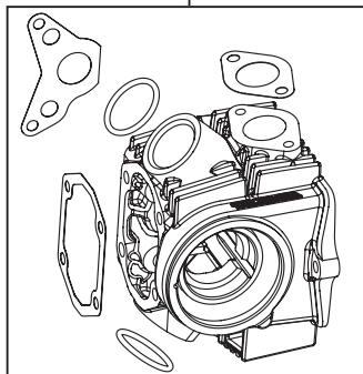
01-03-0023 17R-Stage E ヘッドキット
