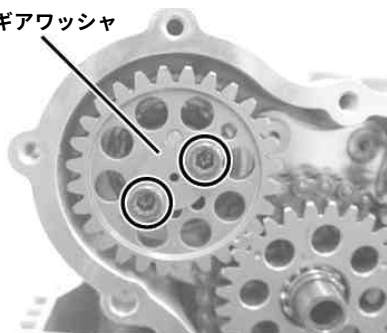
カムギアワッシャ
