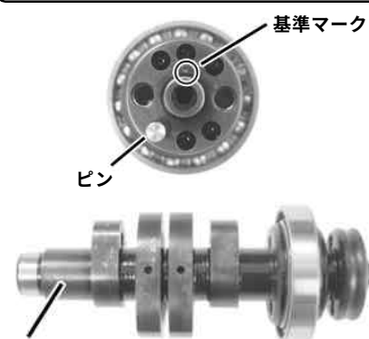
部品番号マーキング位置
