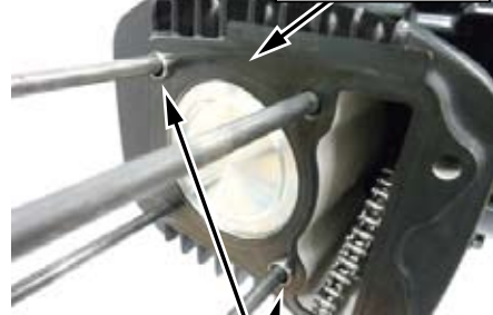
ノックピン
