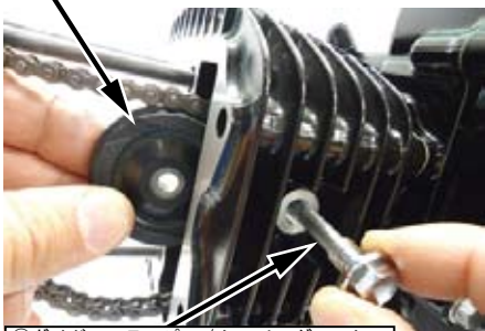
⑪ガイドローラーピン / シーリングワッシャ
