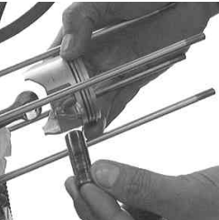
◇ピストンに三分の一程度ピストンピンを挿入しておいて取り付けるのも簡単な方法ではある。 ◇付属のピストンピンサークリップをサークリップ溝にきっちりはめ込む。
