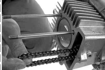
◇カムチェーンを引っ張りながらガイドローラーをつける。
