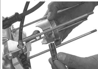
◇ピストンに三分の一程度ピストンピンを挿入しておいて取り付けるのも簡単な方法ではある。 ◇付属のピストンピンサークリップをサークリップ溝にきっちりはめ込む。
