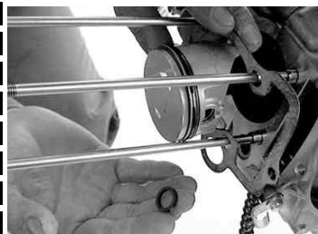
◇シリンダーベースガスケット面のシリンダー側とクランクケース側をシンナー等で脱脂する。
