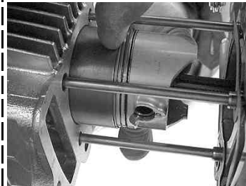
◇シリンダーをピストンリングの合い口がずれないようにしながら指で押し少しずつはめる。ここは難易度が高いです。がんばってください。
