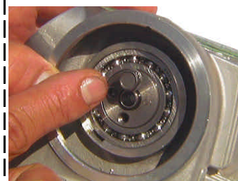
◇カムシャフトにカムスプロケットボルトを取り付け、引っ張るかプラスチックハンマーでヘッドを軽くたたくと抜けてくるので無理に引っ張らずカムシャフトを回しながら取り外す。
