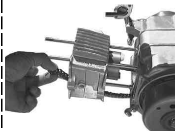
◇リングがシリンダーにはいたらカムチェーンをシリンダーに通しシリンダーをクランクケースにはめる。
