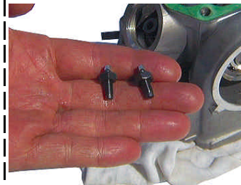
◇カムチェーンを引っ張りながらガイドローラーをつける。
