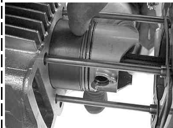
◇シリンダーをピストンリングの合い口がずれないようにしながら指で押し少しずつつはめる。ここは難易度が高いです。がんばってください。
