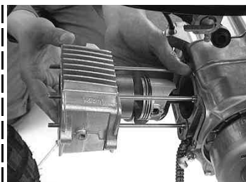
◇タイヤを押さえながらシリンダーを入れていく。
