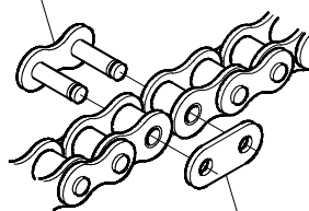
リンクプレート
