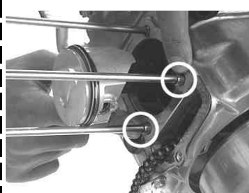
◇ノックピン2個が取り付けられているか点検。
