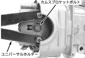
ユニバーサルホルダー
