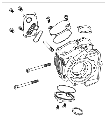
01 03 8005 スーパーヘッド+Rキット
