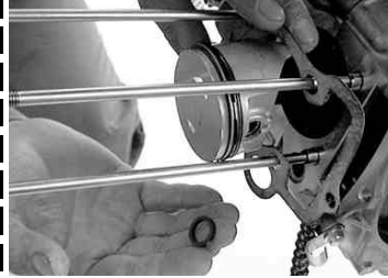
◇シリンダーベースガスケット面のシリンダー側とクランクケース側をシンナー等で脱脂する。
