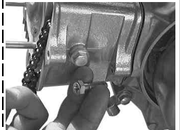
◇シリンダーサイドボルトを取り付ける。（指でしめる程度まで仮止め）
