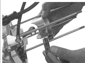
◇ピストンに三分の一程度ピストンピンを挿入しておいて取り付けるのも簡単な方法ではある。 ◇付属のピストンピンサークリップをサークリップ溝にきっちりめ込む。
